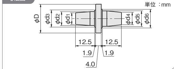
寸法図
