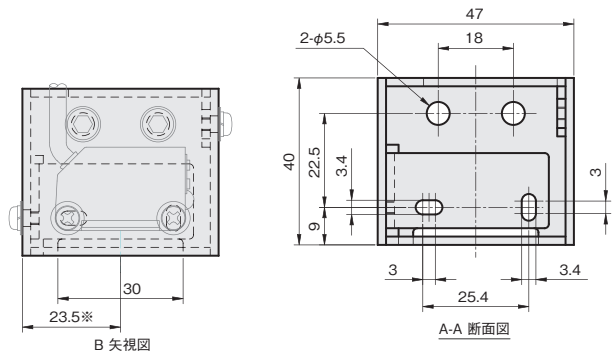
B 矢視図
