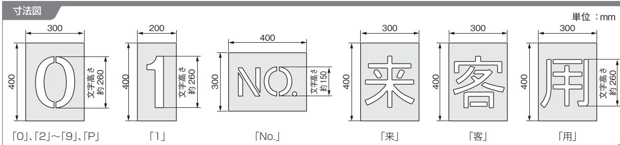
寸法図
