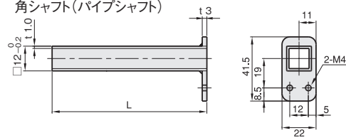
角シャフト(パイプシャフト)
